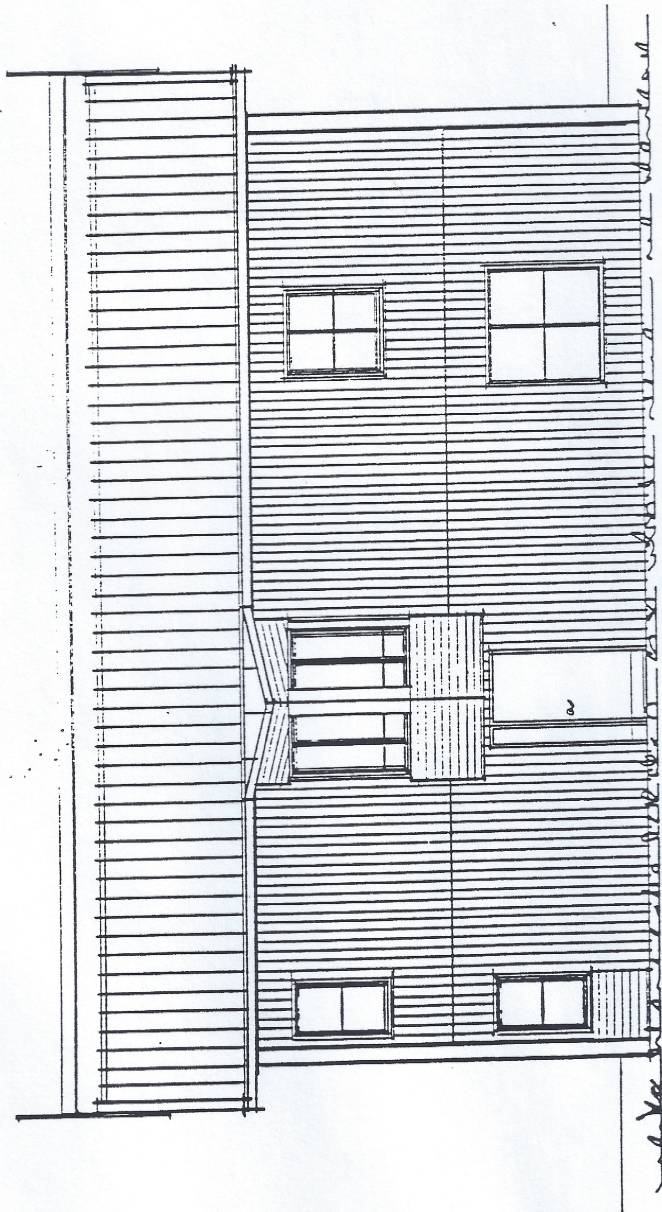
FASAD LÅNGSDA HUSTYP B
